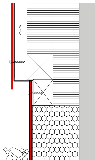
Sockel isoliert (Holzunterkonstruktion)
