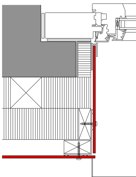
Fensterleibung (Scoba ® glas)
