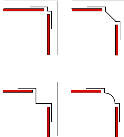
Ausführung von Innenecken
