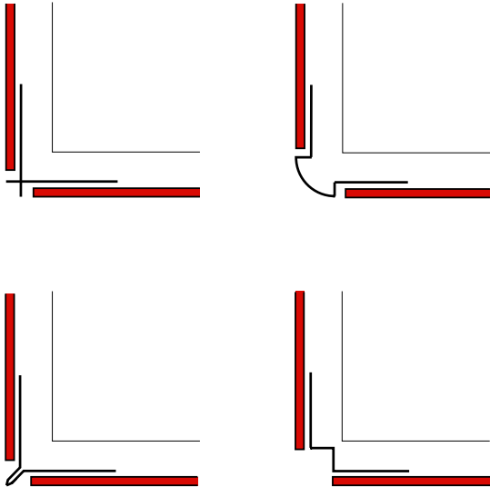
Ausführung von Aussenecken
