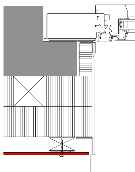
Fensterleibung (Metallabdeckung)
