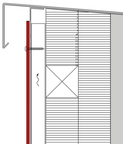
Brüstung
