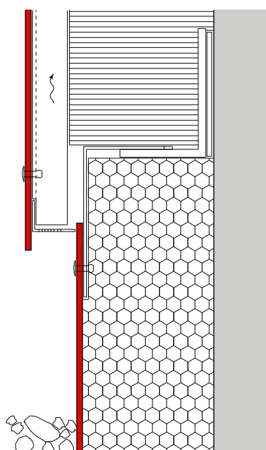
Sockel isoliert (Metallunterkonstruktion)
