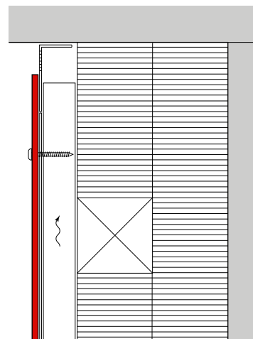
Fassadenabschluss bei Auskrägung
