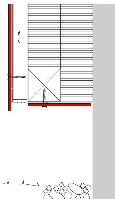
Sockel
